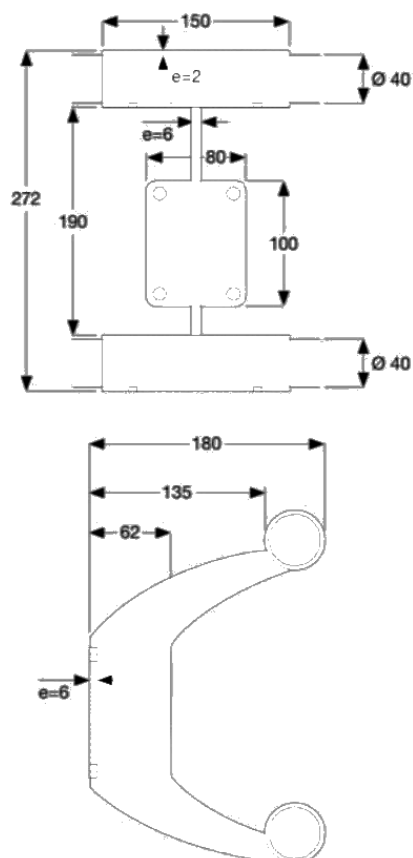
Dessin technique — cotes en mm
