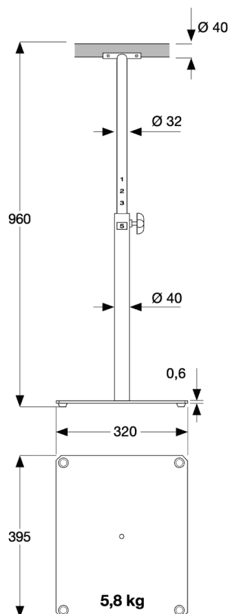
Dessin technique — cotes en mm (épaisseur du socle en cm)
