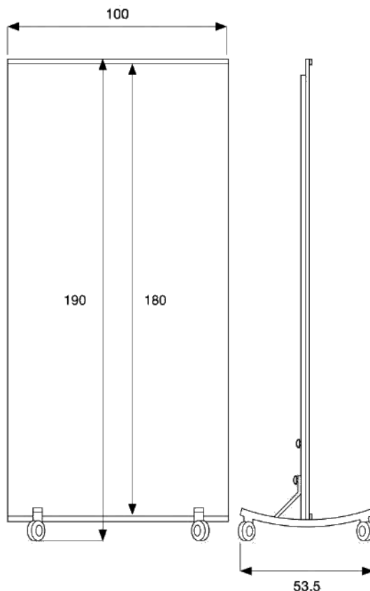
Dessin technique — cotes en cm
