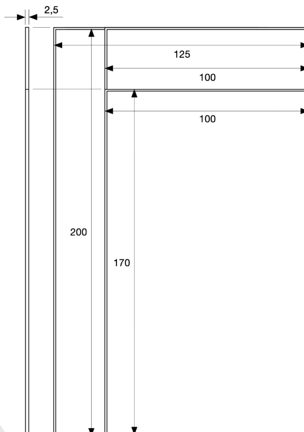
Dessin technique — cotes en cm
