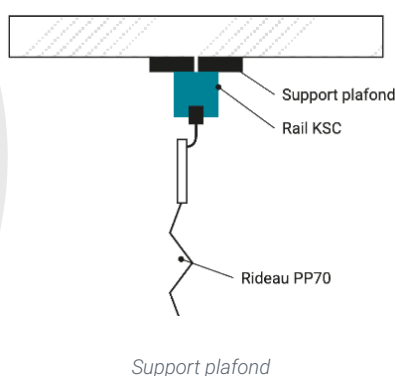
POSE PLAFOND
