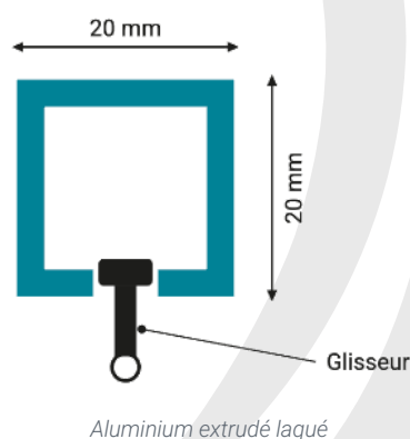
PROFIL KSC
