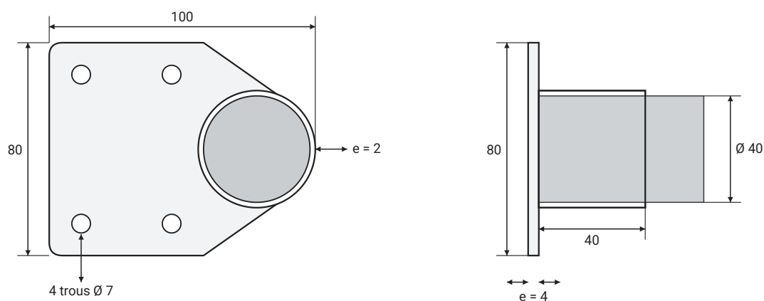
Dessin technique — vue de face et vue de côté, cotes en mm
